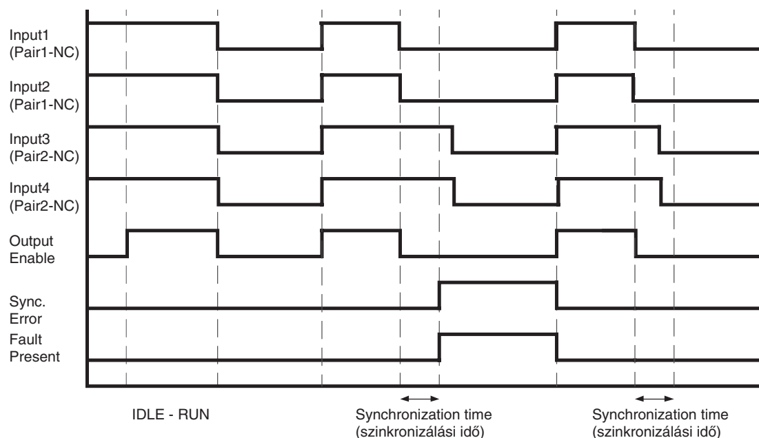
Dual Channel Equivalent (2 Pairs) bemenettípus, működésvizsgálat tiltva
