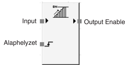
Alapértelmezett kapcsolás
