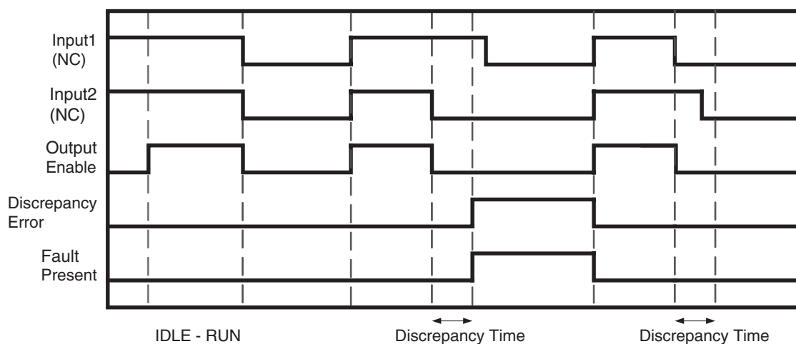
Dual Channel Equivalent (2 Pairs) bemenettípus, működésvizsgálat tiltva
