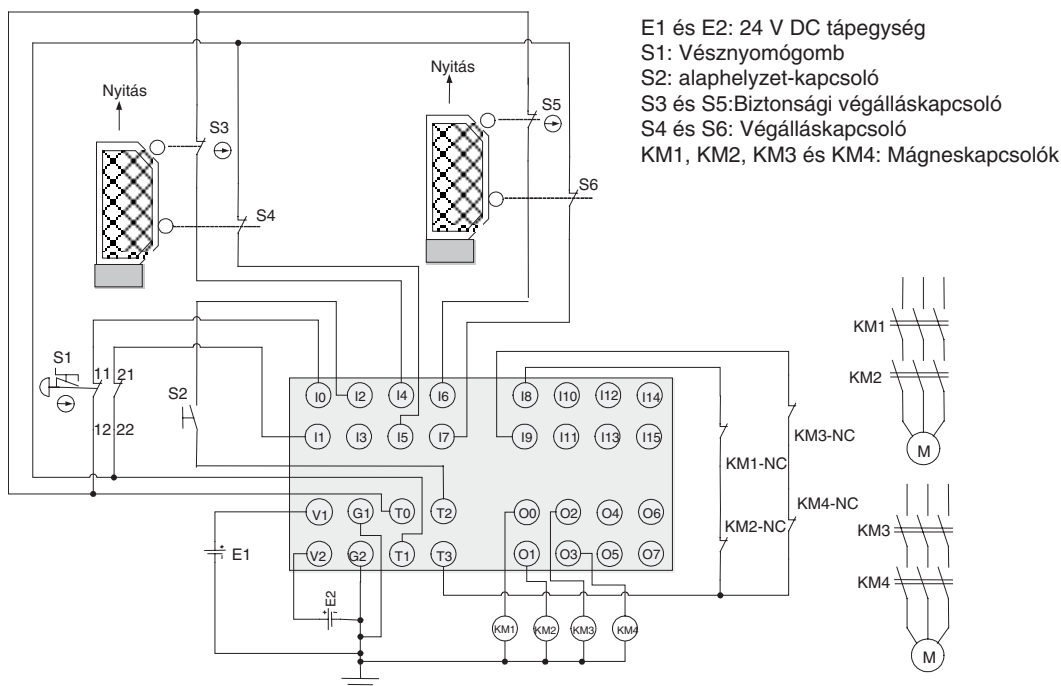
Bekötési rajz
