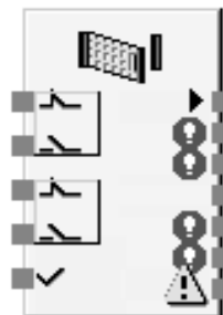
A Biztonsági ajtó monitorozása funkcióblokk megengedett számú bemenet és kimenet engedélyezésével
