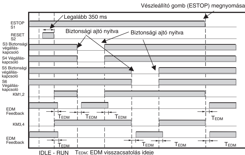
Időzítési diagram
