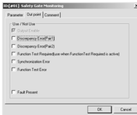
A Biztonsági ajtó monitorozása funkcióblokk szerkesztésére szolgáló párbeszédpanel Out Point panelapja
