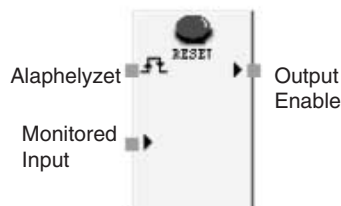
Alapértelmezett kapcsolás
