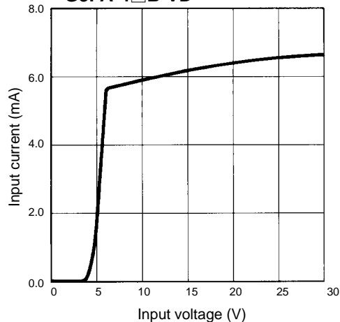
G3PA-4□B-VD
