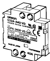
G32A-A40-VD
