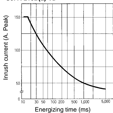
G3PA-420B-VD, G3PA-420B-VD-2
