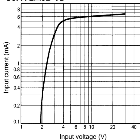
G3PA-2□0B-VD
