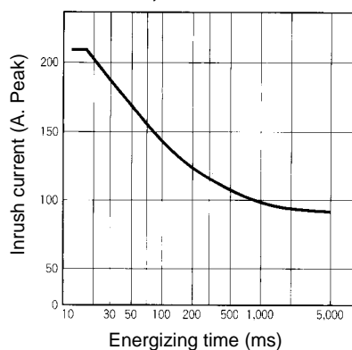
G3PA-420B-VD, G3PA-420B-VD-2
